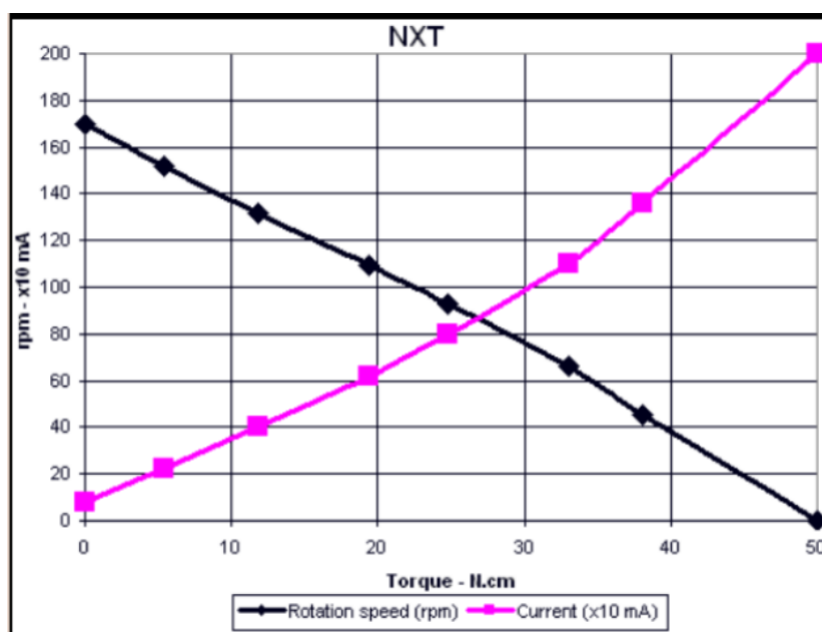
Caractéristiques de vitesse et de courant en fonction du couple utile
